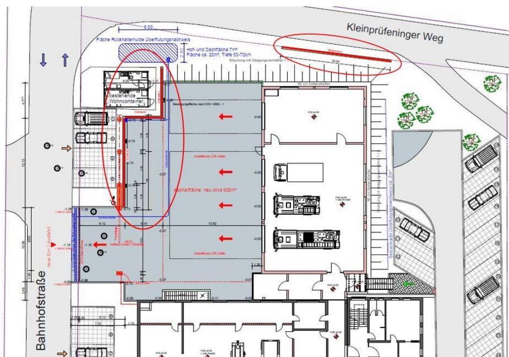
LAGEPLAN
